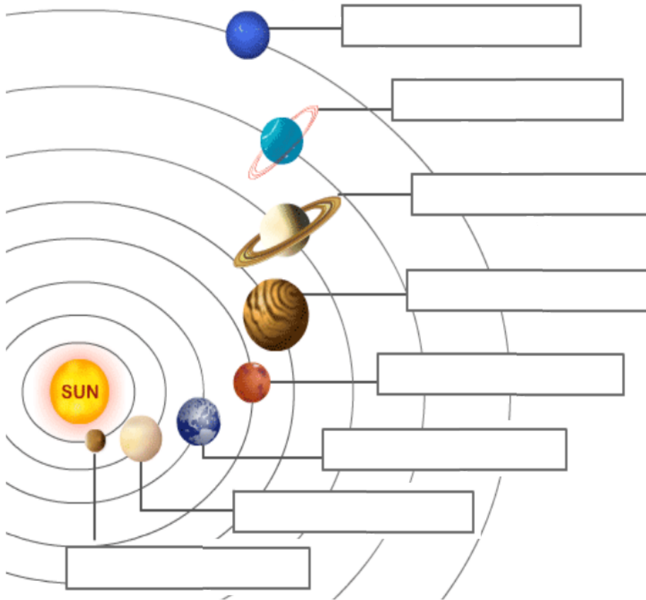
Schéma de l'organisation du système solaire.
